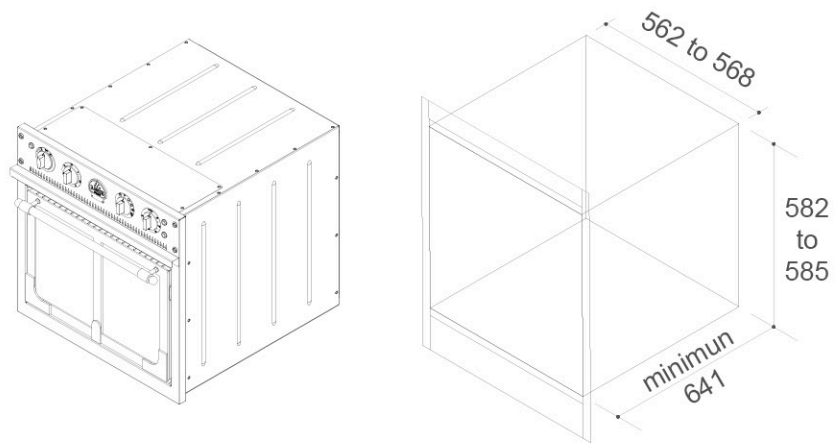
CUTOUT DIMENSIONS
