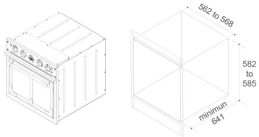
CUTOUT DIMENSIONS
