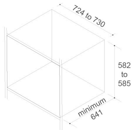
CUTOUT DIMENSIONS
